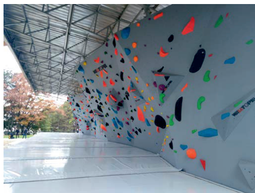
Вештачка стена за спортско пењање Завода за спорт и медицину спорта РС
