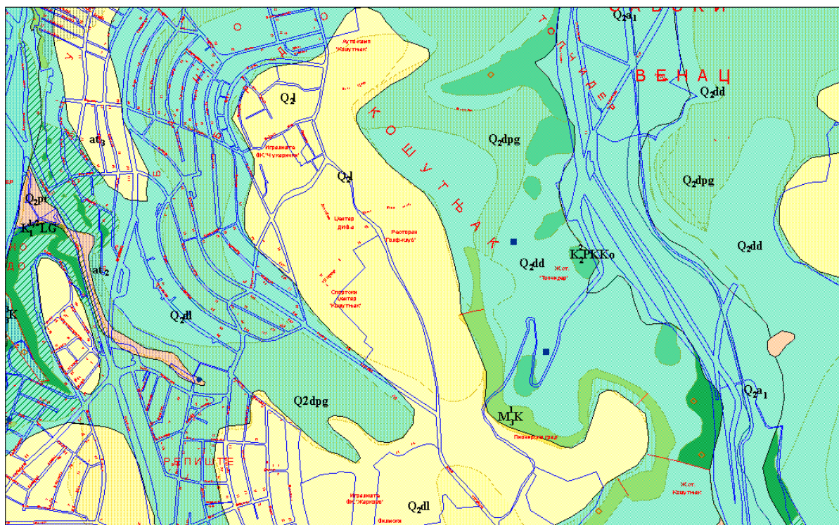
ИНЖЕЊЕРСКОГЕОЛОШКА КАРТА
